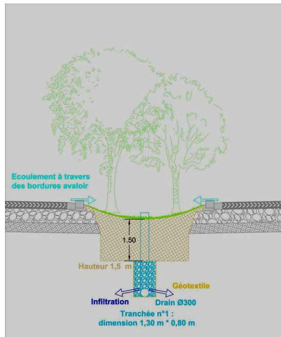
Coupe présentant le principe d'infiltration des eaux
