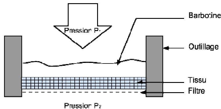
Figure 10 : Schématisation du procédé APS
