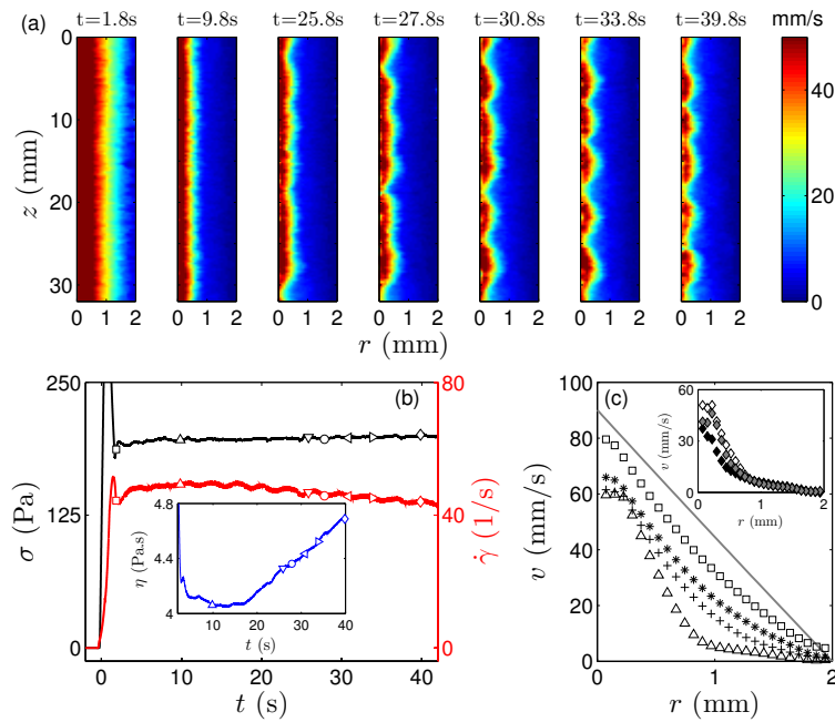
FIGURE 2 – (a) Champ de vitesse v(r, z, t) mesuré par imagerie ultrasonore dans une solution de micelles géantes cisailée à \dot{\gamma} = 40 \pm 4 \text{ s}^{-1} en géométrie de Taylor-Couette cylindrique d’entrefer 2 mm. r correspond à la distance au cylindre intérieur tournant et z à la position verticale. (b) Réponses rhéologiques \dot{\gamma}(t) (en noir), \sigma(t) (en rouge) et \eta(t) (insert, en bleu). (c) Profils de vitesse moyennés selon z à t = 1.8 ( \square ), 2.3 ( * ), 2.8 ( + ) et 9.8 s ( \triangle ). La droite grise montre le profil attendu pour un fluide newtonien. Insert : profils de vitesse v(r, z, t) à t = 39.8 s pour différentes positions verticales z = 10.5 (blanc), 9.5 (gris) et 8.5 mm (noir). Figure extraite de [16].
