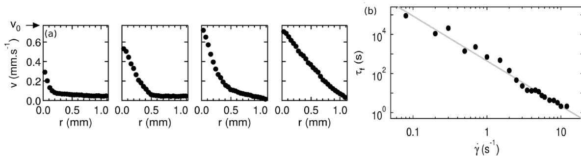
FIGURE 3 – (a) Profils de vitesse v(r, t) mesurés par vélocimétrie ultrasonore dans un microgel de carbopol cisailé à \dot{\gamma} = 0.7 \text{ s}^{-1} en géométrie de Taylor-Couette cylindrique d'entrefer 1 mm pour t = 27, 1013, 1730 et 9413 \text{ s} de gauche à droite. v_0 indique la vitesse du rotor et r correspond à la distance au cylindre intérieur tournant. (b) Temps de fluidification totale \tau_f vs \dot{\gamma} . L'ajustement en gris est \tau_f \sim \dot{\gamma}^{-2/3} .
