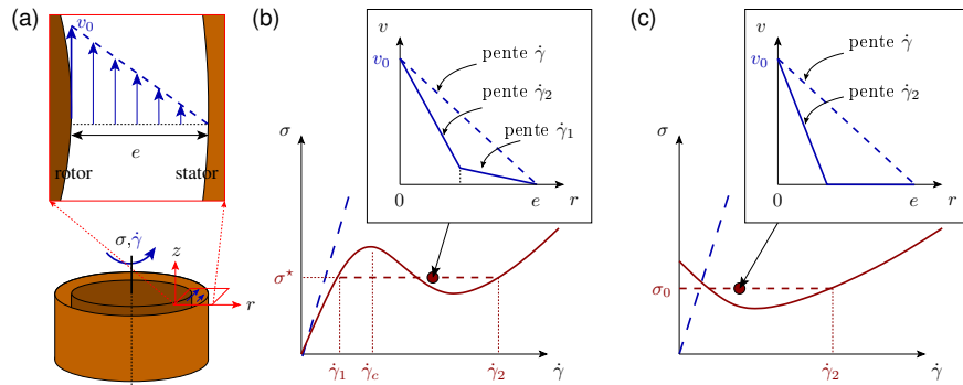
FIGURE 1 – (a) Cisaillement en géométrie de Taylor-Couette et notations utilisées. Courbes d'écoulement \sigma vs \dot{\gamma} et profils de vitesse v(r) attendus pour (b) une solution de micelles géantes et (c) un fluide à seuil présentant des bandes de cisaillement à l'état stationnaire. Les pointillés bleus indiquent le cas d'un fluide newtonien.
