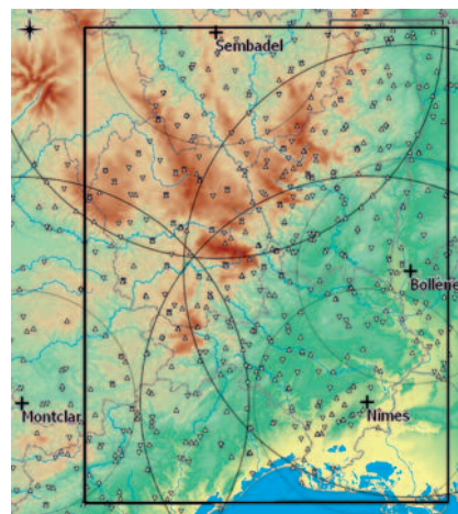
Figure 1. Fenêtre d'observation de l'OHM-CV. Le système d'observation opérationnel des pluies est représenté : pluviographes ( \Delta ), pluviomètres ( \nabla ), radars (+ et marqueurs de distance à 50 et 100 km).
