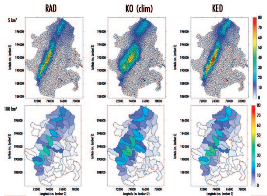
Figure 5. Exemple d'un champ pluvieux horaire observé lors de l'épisode des 19-22 octobre 2008 (entre 21:00 et 22:00 TU le 21), avec, à gauche, l'estimation radar, au centre, l'estimation issue du réseau pluviographique par krigeage ordinaire et, à droite, celle issue de la fusion radar-pluviomètre par krigeage avec dérive externe. Les graphes du haut correspondent au « maillage hydrologique » de 5 km 2 et ceux du bas à celui de 100 km 2 . Le domaine d'estimation couvre les bassins versants de l'Ardèche, de la Cèze, des Gardons et du Vidourle.
