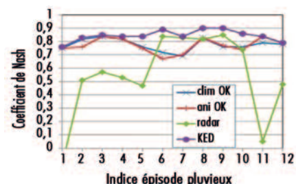
Figure 4. À gauche : liste des 12 épisodes sélectionnés en 2008, avec indication des altitudes minimales et maxi-males de l'isotherme 0 °C déterminé à l'aide des radiosondages de Nîmes. À droite : évolution pour les différents épisodes du coefficient de Nash entre valeurs estimées et observées (validation croisée) au pas de temps horaire, pour les quatre méthodes d'estimation présentées dans le texte.
