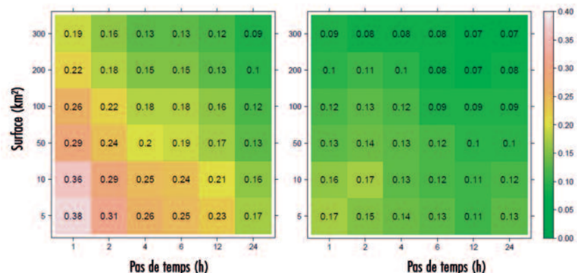
Figure 7. Valeurs moyennes des écart types d'erreur normés par l'estimation de pluie pour les estimations issues du krigeage ordinaire (à gauche) et du krigeage avec dérive externe (à droite) en fonction des pas de temps et d'espace considérés, pour les épisodes 6 à 10.
