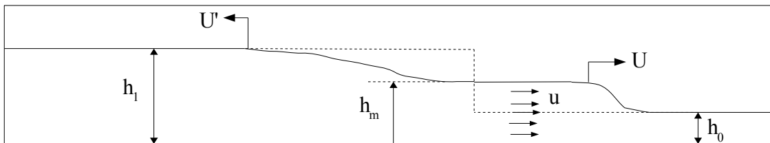
FIG. 1 – Schématisation d'un lâcher de barrage sur fond plat.
